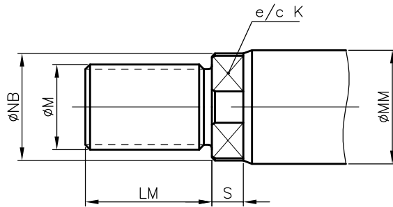
Roscado exterior – 1
